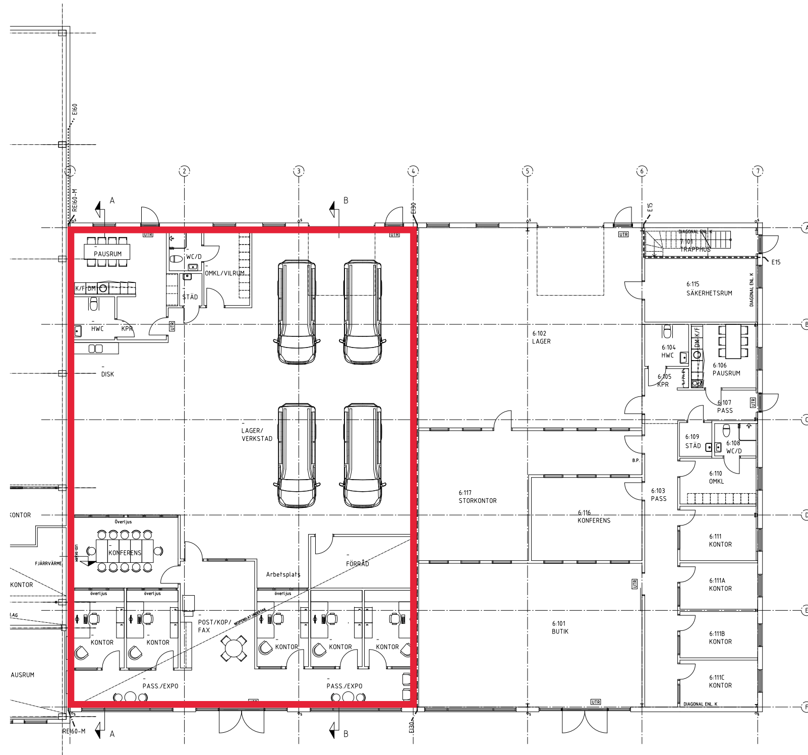
PLAN 1 SKALA 1:100
