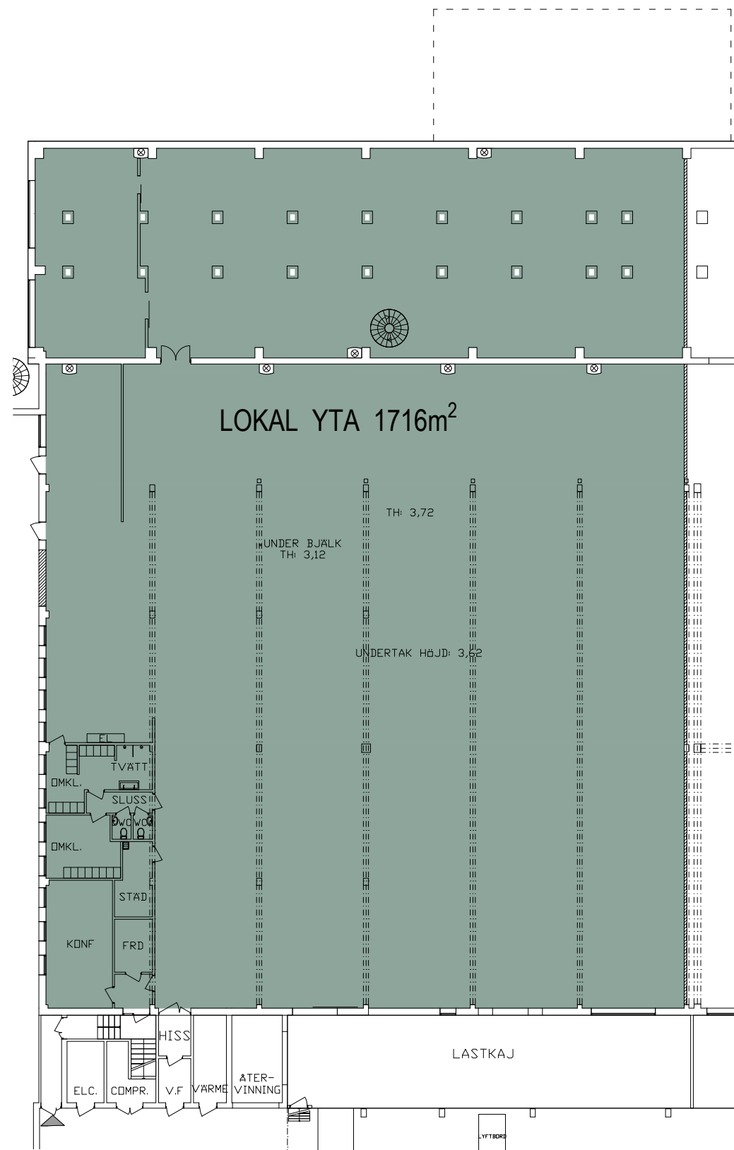
PLAN 0 SKALA 1:300 i A3
