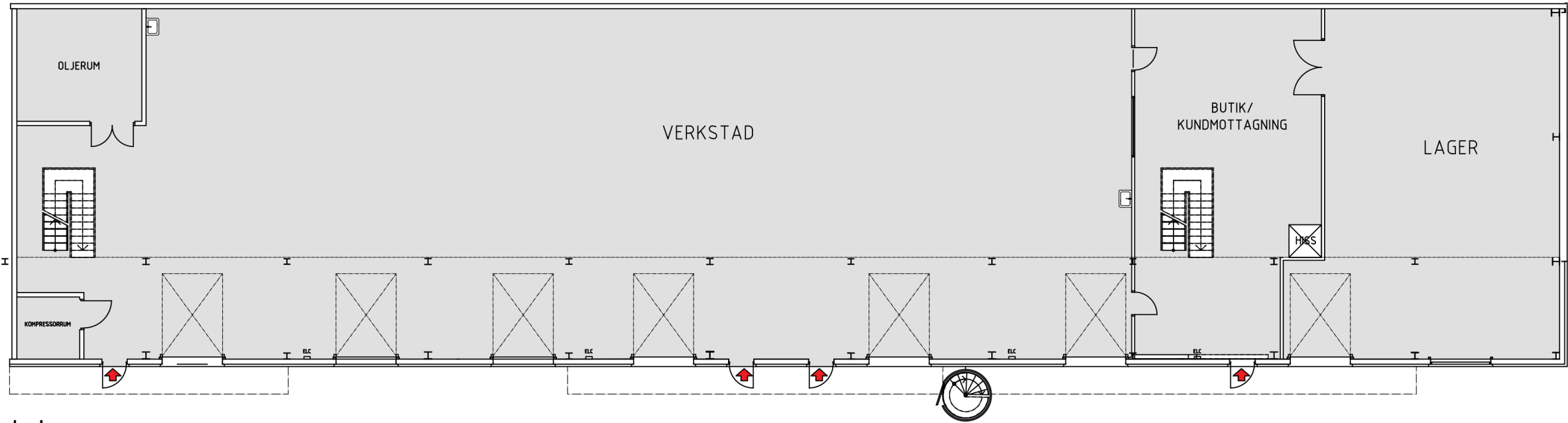
Markplan Lager, Verkstad, mm. - ca 832 kvm
