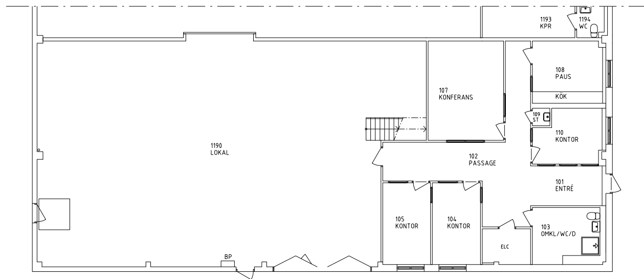
BOTTENVÅNING, DELPLAN 1:200
