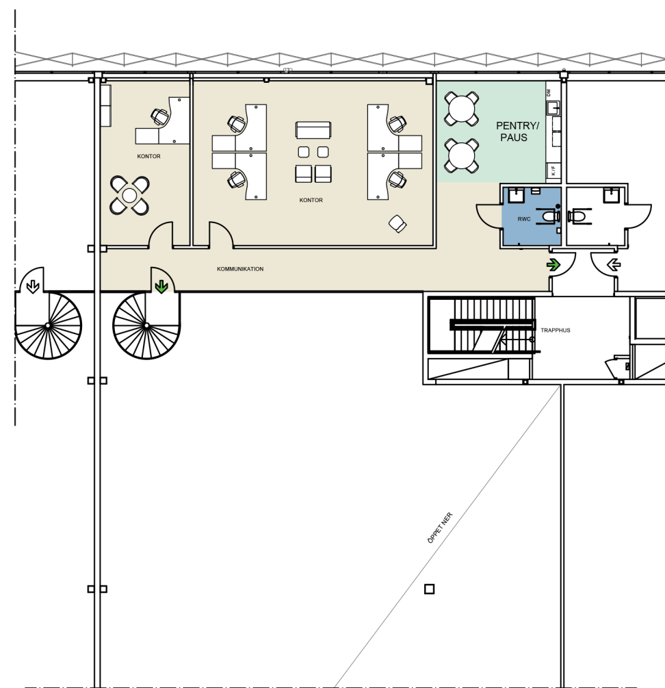
Entrésolplan Kontor
